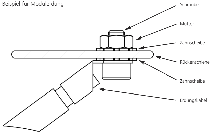
Beispiel für Modulerdung
