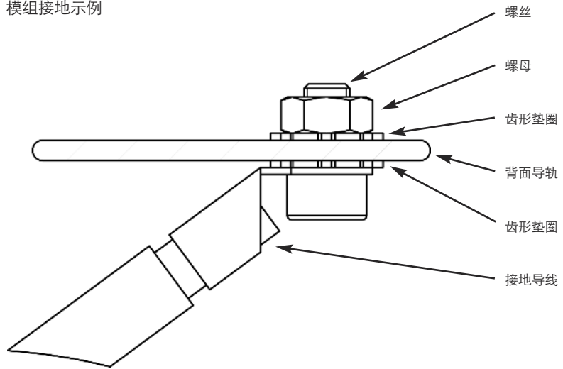
模组接地示例
